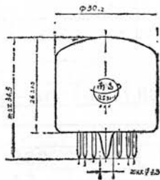
外形图：
