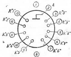
电极接线图
