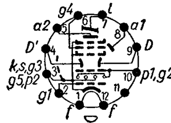
Sockelschaltenschema
